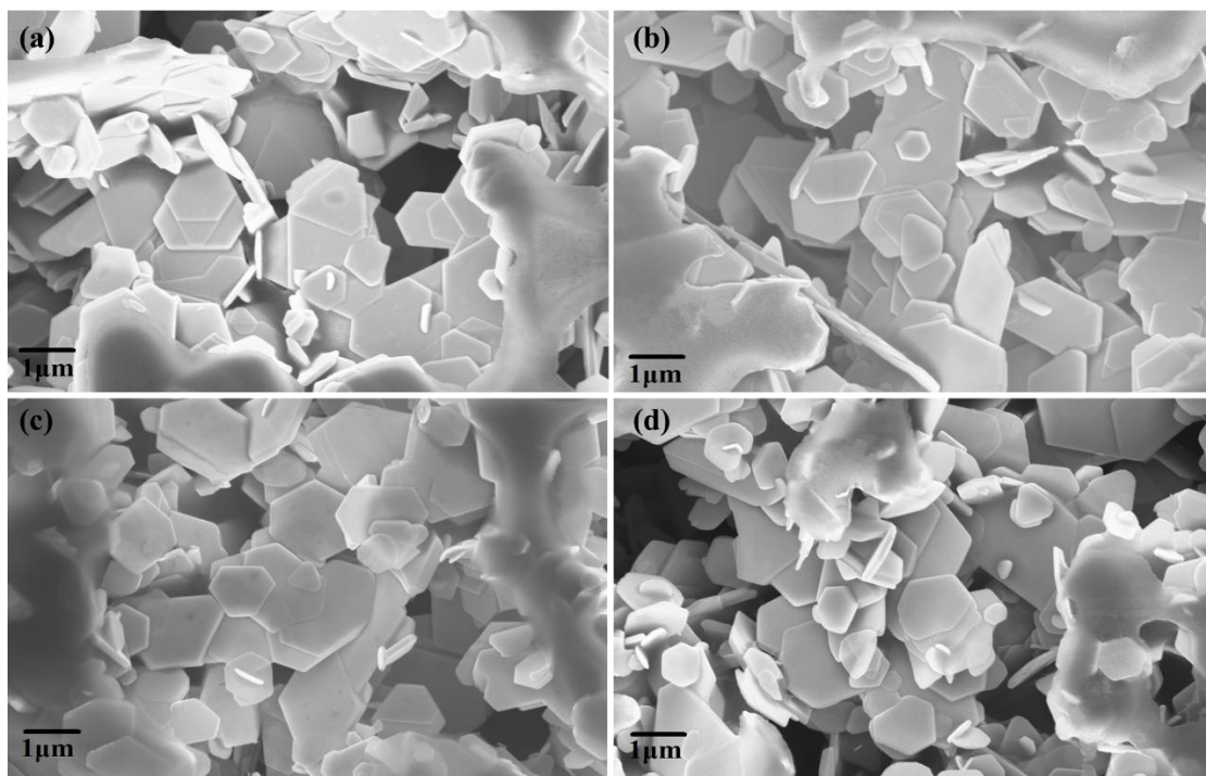
Fig. S3. Flat SEM images of \text{Bi}_2\text{Se}_{3+x} /PVDF composite films: (a) x=0 , (b) x=0.2 , (c) x=0.3 and (d) x=0.4 .
