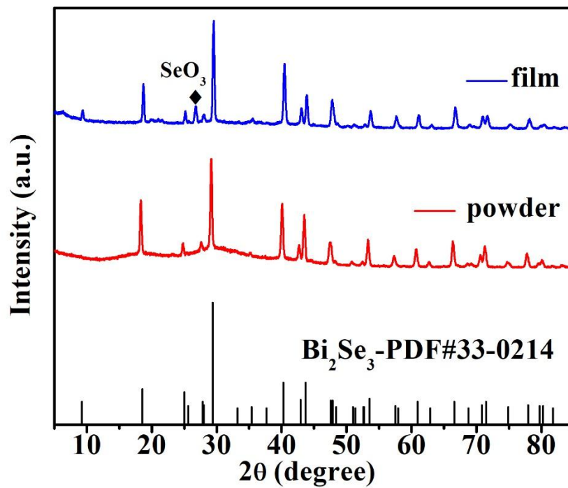
Fig. S1. XRD patterns of Bi 2 Se 3.2 /PVDF composite films and Bi 2 Se 3.2 powder.
